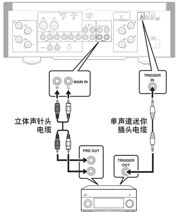
Yamaha AV 接收器或其他带有 TRIGGER OUT 插孔和 PRE OUT 插孔的组件
