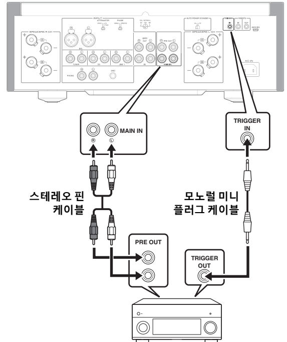
Yamaha AV 리시버 또는 TRIGGER OUT 잭과 PRE OUT 잭이 있는 기타 컴포넌트
